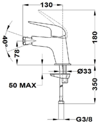
Grifo de bidé • Rótula orientable • Aireador antical • Conexiones flexibles 3/8"-1/2" incluidas • Sin desagüe automático
