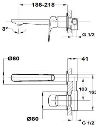
Grifo de lavabo Mural • Aireador antical
