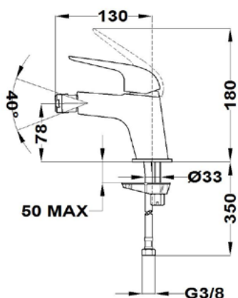
Grifo de bidé • Rótula orientable • Aireador antical • Conexiones flexibles 3/8"-1/2" incluidas • Sin desagüe automático • Acabado Metallic (PVD) • Tratamiento anti-huellas en acabados Metallic (PVD)
